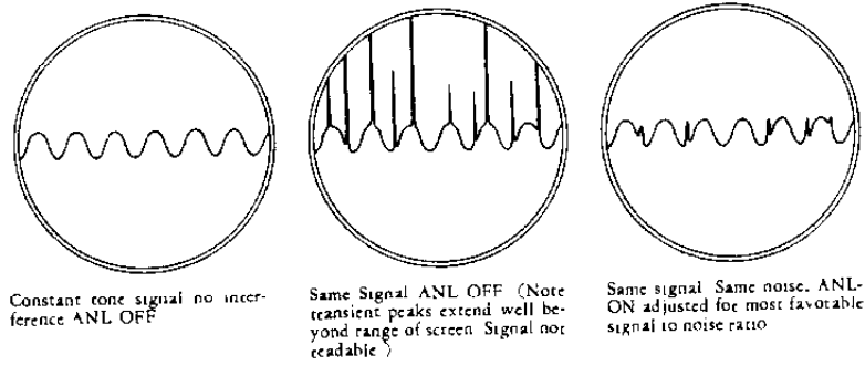
FIG. 6—NOISE LIMITER ACTION
